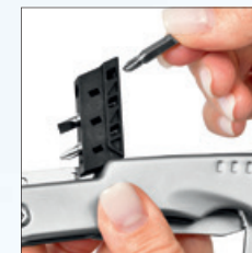
integrierter Bithalter
